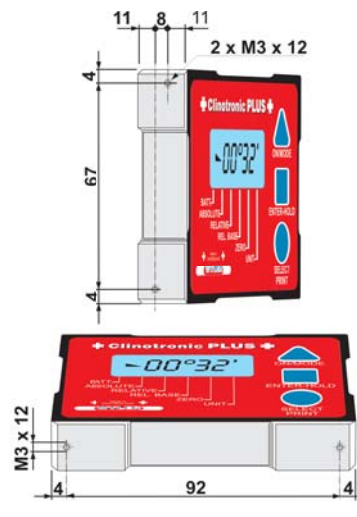
Linke Abbildung: +CLINO PLUS+ mit Magneteinsätzen links und unten / z.B. 015-PLUS-FG45 Rechte Abbildung: +CLINO PLUS+ Gewinden M3 links und unten / z.B. 015-PLUS-LG45
